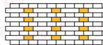
Голландская кладка
